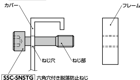
SSC-SNSTG 六角穴付き脱落防止ねじ
